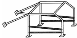
Dessin / Drawing N°253-17
