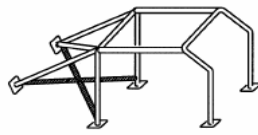
Dessin / Drawing N°253-15
