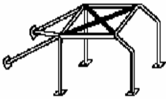
Dessin / Drawing N° 253-9
