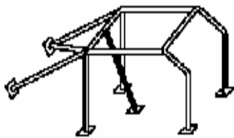
Dessin / Drawing N° 253-6
