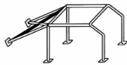
Dessin / Drawing N°253-17A
